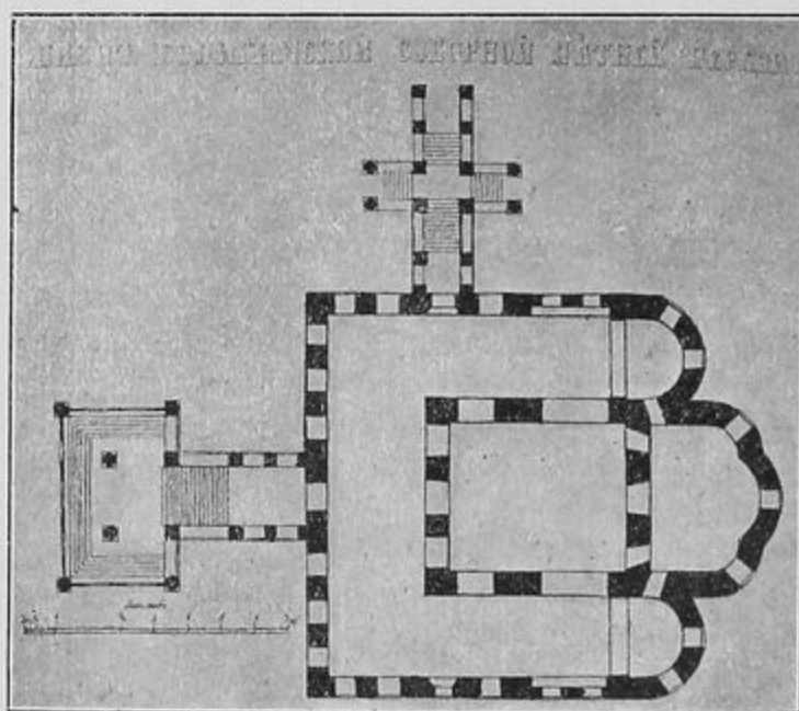
Рис. 1. Святотроицкій лѣтній соборъ.
